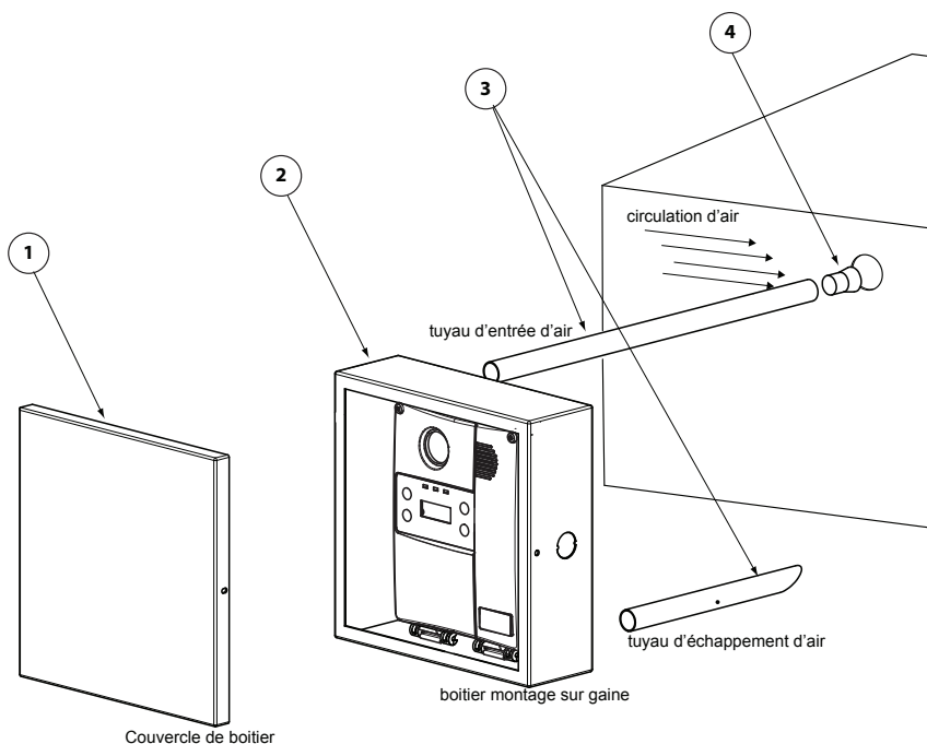
Illustration 8. Pièce pour montage sur gaine
