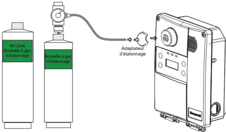
Illustration 6. Installation d'étalonnage
