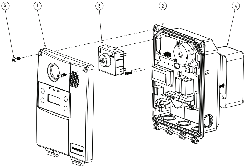
Illustration 7. Pièces du E 3 Point
